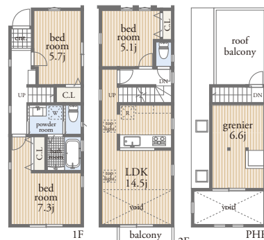
LDK(A号棟)
